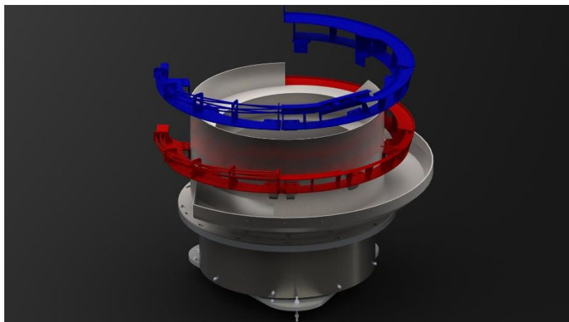
Verschiedene Formatsätze für den 630er Zylindertopf
